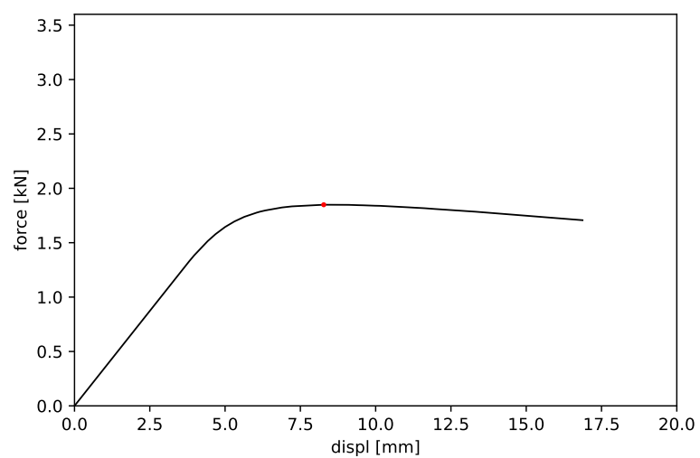
Obrázek 27: Vzorek č. 27 - maximální síla 1.849 kN a příslušný posun 8.276 mm
