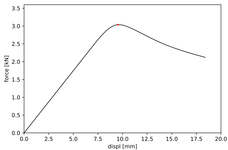
Obrázek 40: Vzorek č. 40 - maximální síla 3.039 kN a příslušný posun 9.537 mm
