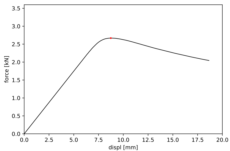
Obrázek 46: Vzorek č. 46 - maximální síla 2.669 kN a příslušný posun 8.741 mm
