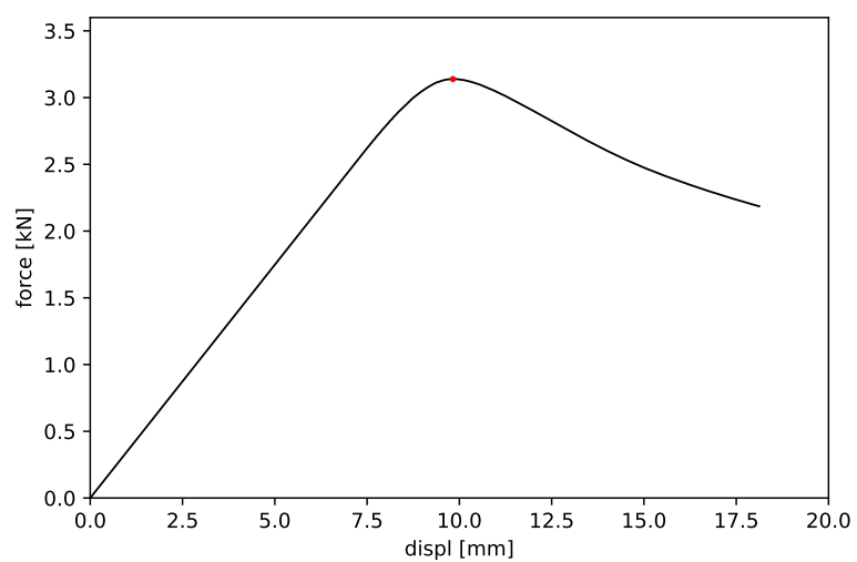
Obrázek 61: Vzorek č. 61 - maximální síla 3.139 kN a příslušný posun 9.826 mm
