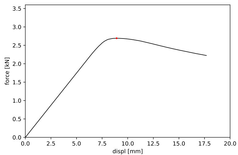
Obrázek 14: Vzorek č. 14 - maximální síla 2.692 kN a příslušný posun 8.916 mm
