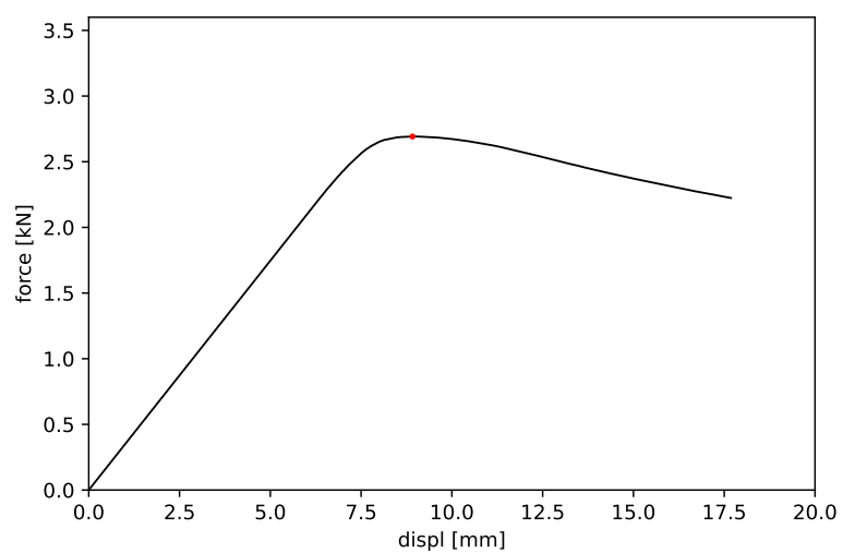
Obrázek 15: Vzorek č. 15 - maximální síla 2.692 kN a příslušný posun 8.916 mm
