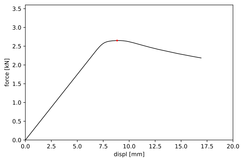
Obrázek 10: Vzorek č. 10 - maximální síla 2.651 kN a příslušný posun 8.835 mm
