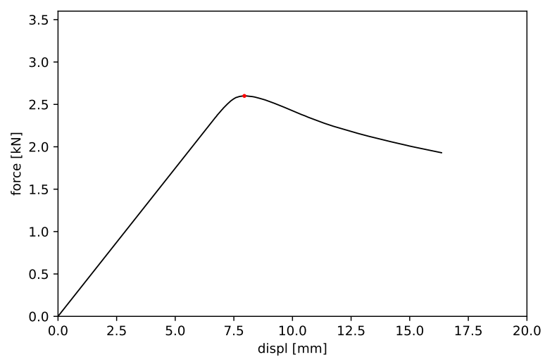
Obrázek 34: Vzorek č. 34 - maximální síla 2.600 kN a příslušný posun 7.949 mm
