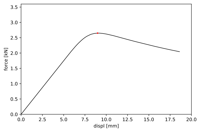
Obrázek 21: Vzorek č. 21 - maximální síla 2.650 kN a příslušný posun 8.983 mm
