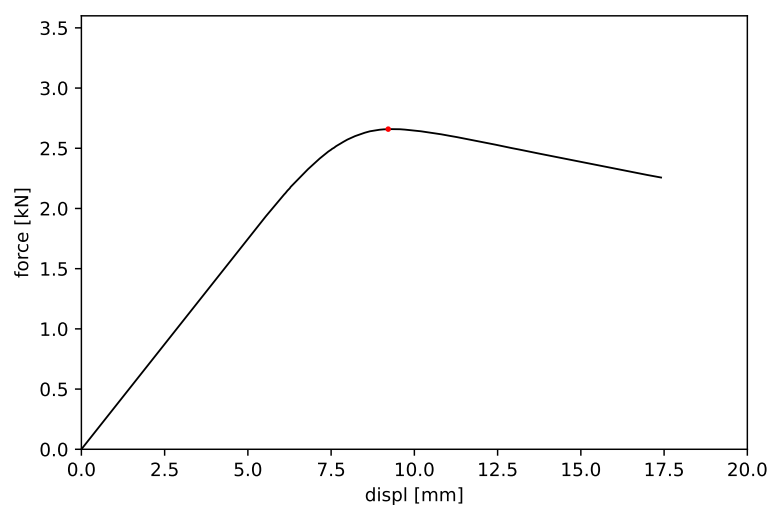
Obrázek 35: Vzorek č. 35 - maximální síla 2.659 kN a příslušný posun 9.215 mm
