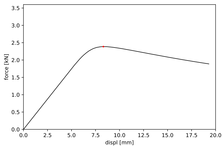
Obrázek 56: Vzorek č. 56 - maximální síla 2.387 kN a příslušný posun 8.317 mm
