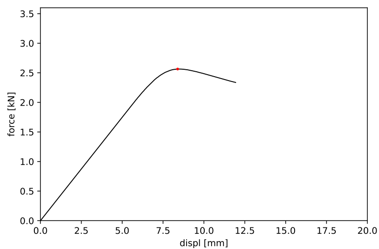
Obrázek 12: Vzorek č. 12 - maximální síla 2.564 kN a příslušný posun 8.392 mm
