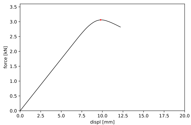
Obrázek 30: Vzorek č. 30 - maximální síla 3.062 kN a příslušný posun 9.785 mm
