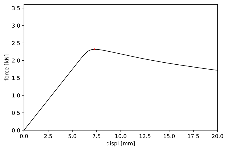
Obrázek 13: Vzorek č. 13 - maximální síla 2.319 kN a příslušný posun 7.288 mm
