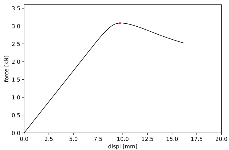
Obrázek 33: Vzorek č. 33 - maximální síla 3.084 kN a příslušný posun 9.721 mm
