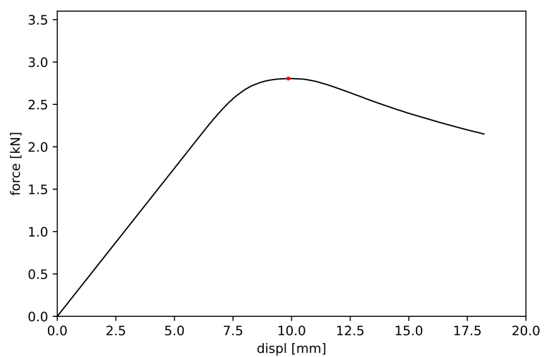
Obrázek 57: Vzorek č. 57 - maximální síla 2.805 kN a příslušný posun 9.863 mm
