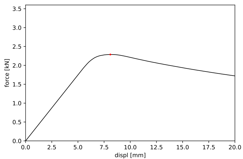
Obrázek 41: Vzorek č. 41 - maximální síla 2.288 kN a příslušný posun 8.096 mm
