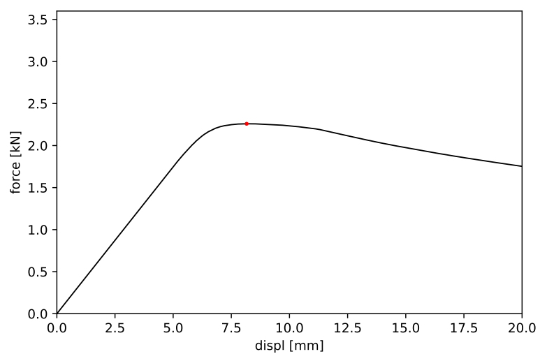
Obrázek 5: Vzorek č. 5 - maximální síla 2.259 kN a příslušný posun 8.157 mm
