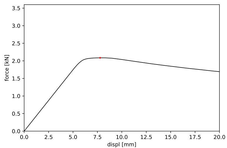
Obrázek 11: Vzorek č. 11 - maximální síla 2.086 kN a příslušný posun 7.777 mm
