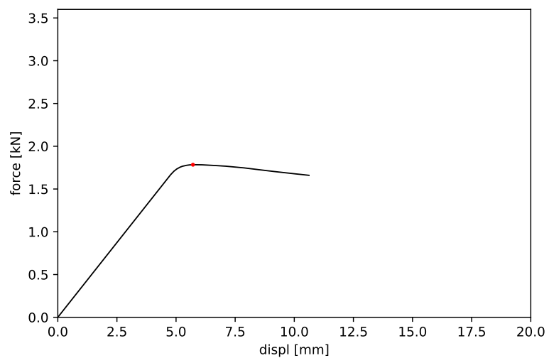
Obrázek 1: Vzorek č. 1 - maximální síla 1.784 kN a příslušný posun 5.714 mm
