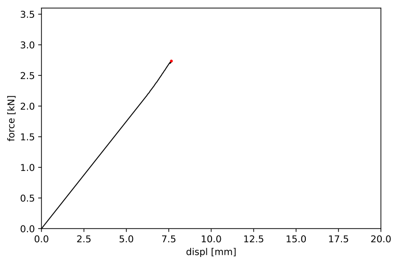
Obrázek 22: Vzorek č. 22 - maximální síla 2.735 kN a příslušný posun 7.654 mm
