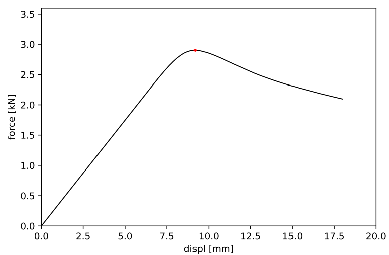
Obrázek 9: Vzorek č. 9 - maximální síla 2.900 kN a příslušný posun 9.185 mm
