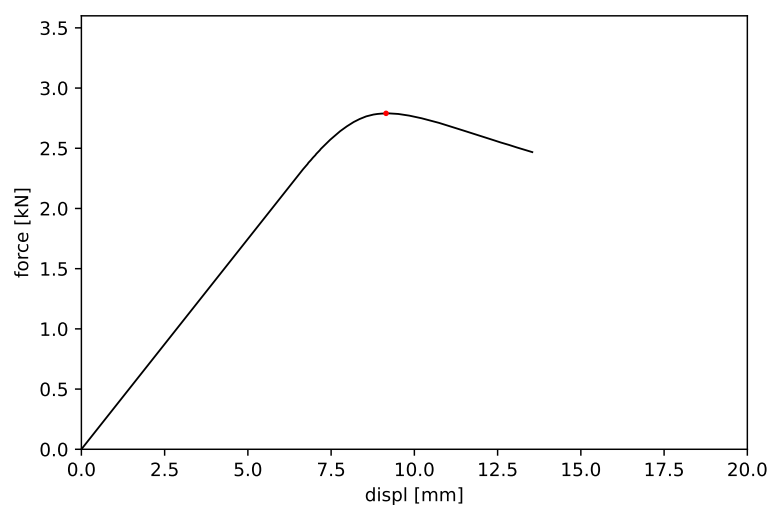
Obrázek 31: Vzorek č. 31 - maximální síla 2.790 kN a příslušný posun 9.150 mm
