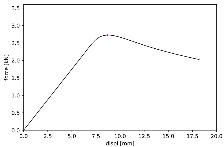
Obrázek 37: Vzorek č. 37 - maximální síla 2.726 kN a příslušný posun 8.699 mm
