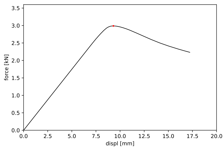
Obrázek 8: Vzorek č. 8 - maximální síla 2.989 kN a příslušný posun 9.309 mm
