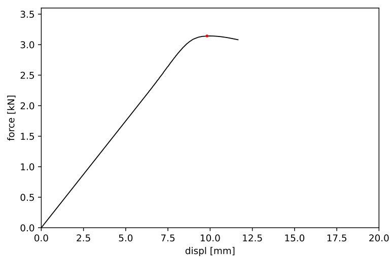
Obrázek 17: Vzorek č. 17 - maximální síla 3.142 kN a příslušný posun 9.817 mm
