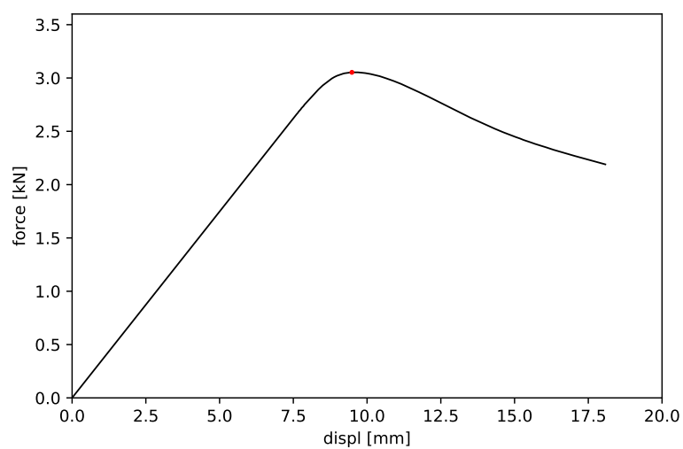
Obrázek 48: Vzorek č. 48 - maximální síla 3.053 kN a příslušný posun 9.486 mm
