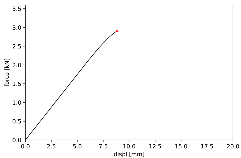
Obrázek 51: Vzorek č. 51 - maximální síla 2.904 kN a příslušný posun 8.827 mm
