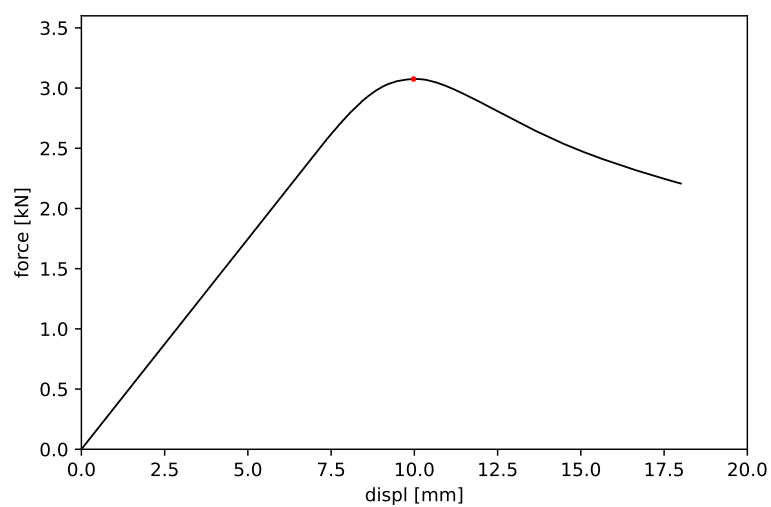
Obrázek 42: Vzorek č. 42 - maximální síla 3.075 kN a příslušný posun 9.977 mm
