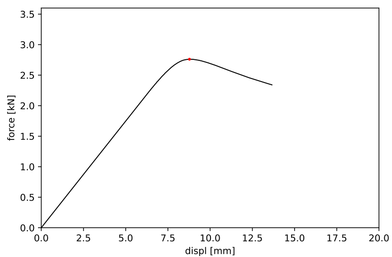
Obrázek 53: Vzorek č. 53 - maximální síla 2.761 kN a příslušný posun 8.777 mm
