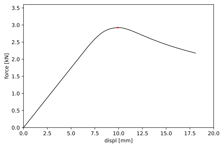
Obrázek 44: Vzorek č. 44 - maximální síla 2.924 kN a příslušný posun 9.925 mm
