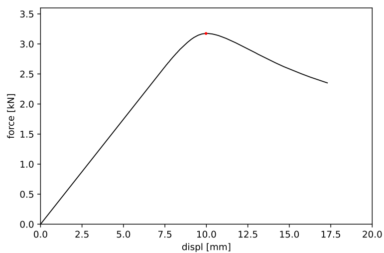
Obrázek 60: Vzorek č. 60 - maximální síla 3.174 kN a příslušný posun 9.978 mm
