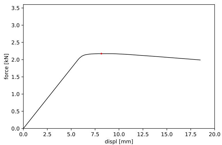
Obrázek 6: Vzorek č. 6 - maximální síla 2.174 kN a příslušný posun 8.157 mm
