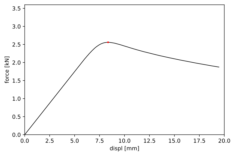
Obrázek 20: Vzorek č. 20 - maximální síla 2.560 kN a příslušný posun 8.354 mm
