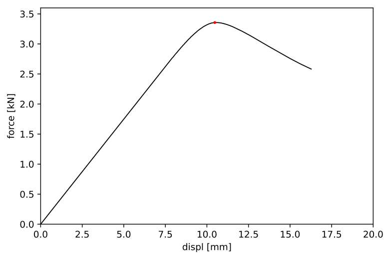
Obrázek 64: Vzorek č. 64 - maximální síla 3.356 kN a příslušný posun 10.474 mm
