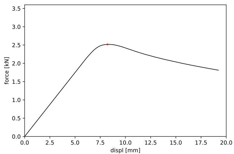
Obrázek 2: Vzorek č. 2 - maximální síla 2.517 kN a příslušný posun 8.210 mm
