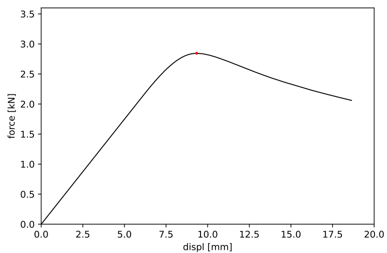
Obrázek 23: Vzorek č. 23 - maximální síla 2.844 kN a příslušný posun 9.341 mm
