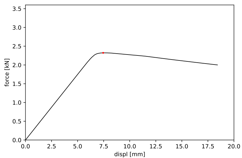
Obrázek 4: Vzorek č. 4 - maximální síla 2.323 kN a příslušný posun 7.451 mm
