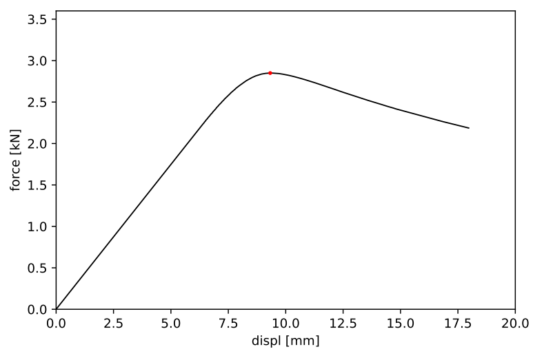
Obrázek 58: Vzorek č. 58 - maximální síla 2.850 kN a příslušný posun 9.325 mm
