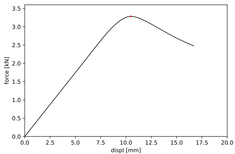
Obrázek 50: Vzorek č. 50 - maximální síla 3.283 kN a příslušný posun 10.447 mm
