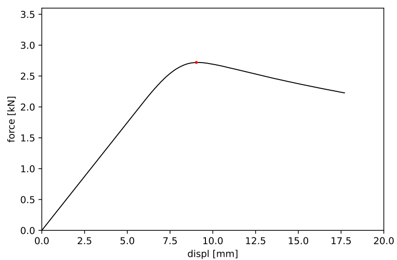
Obrázek 43: Vzorek č. 43 - maximální síla 2.720 kN a příslušný posun 9.037 mm
