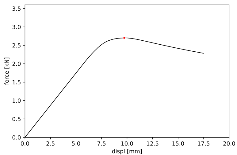
Obrázek 19: Vzorek č. 19 - maximální síla 2.701 kN a příslušný posun 9.719 mm
