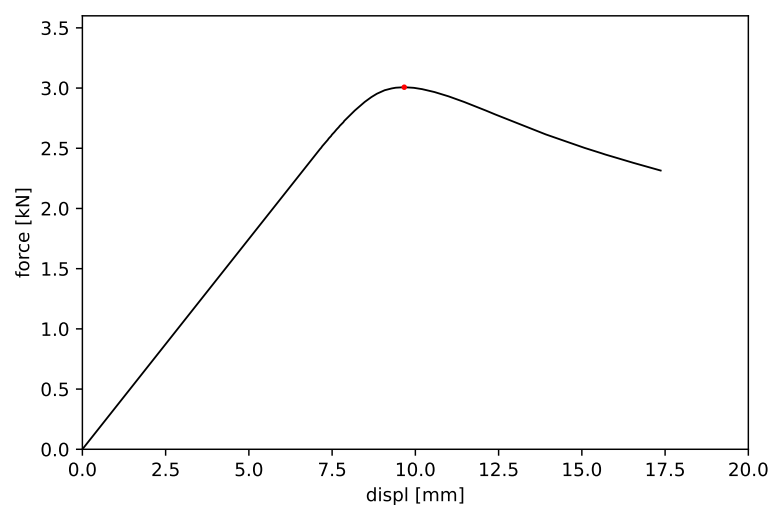
Obrázek 49: Vzorek č. 49 - maximální síla 3.007 kN a příslušný posun 9.666 mm
