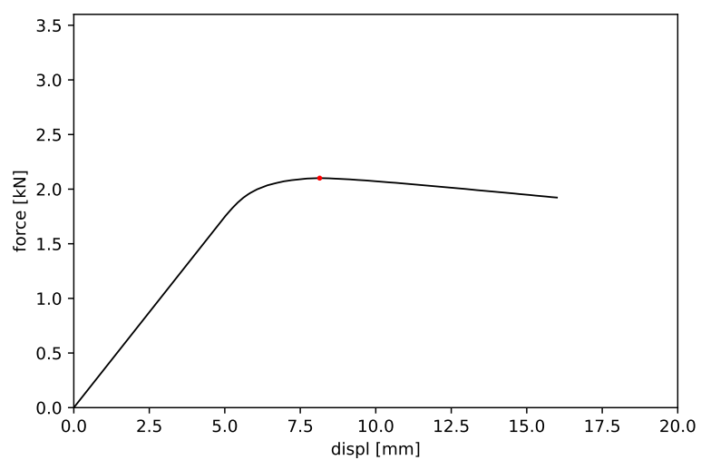
Obrázek 29: Vzorek č. 29 - maximální síla 2.101 kN a příslušný posun 8.142 mm
