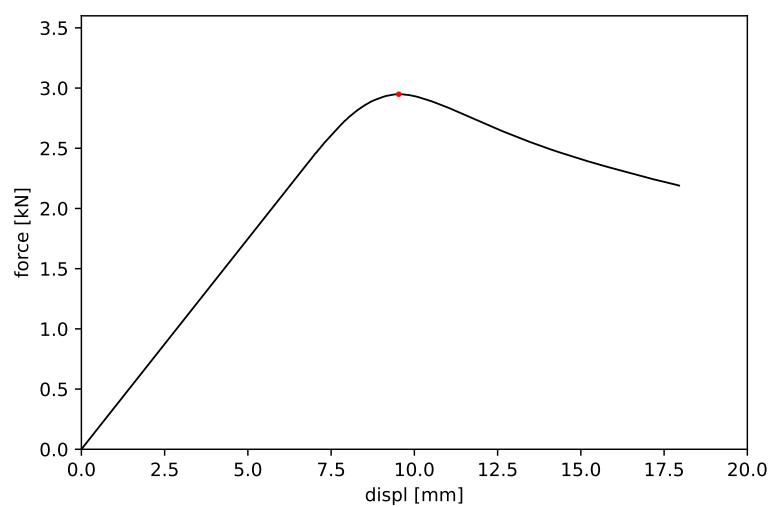
Obrázek 25: Vzorek č. 25 - maximální síla 2.949 kN a příslušný posun 9.531 mm
