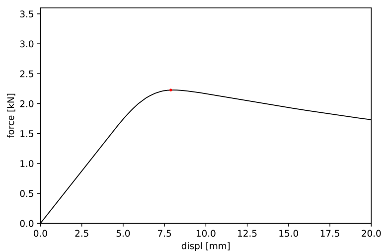
Obrázek 18: Vzorek č. 18 - maximální síla 2.227 kN a příslušný posun 7.882 mm
