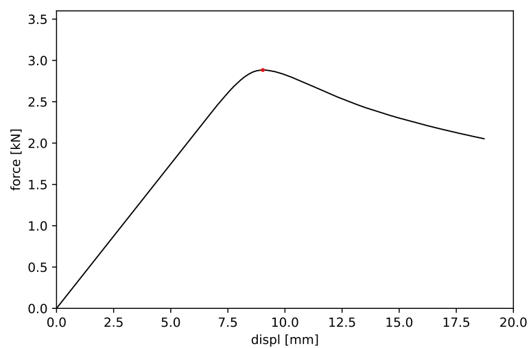
Obrázek 62: Vzorek č. 62 - maximální síla 2.884 kN a příslušný posun 9.033 mm
