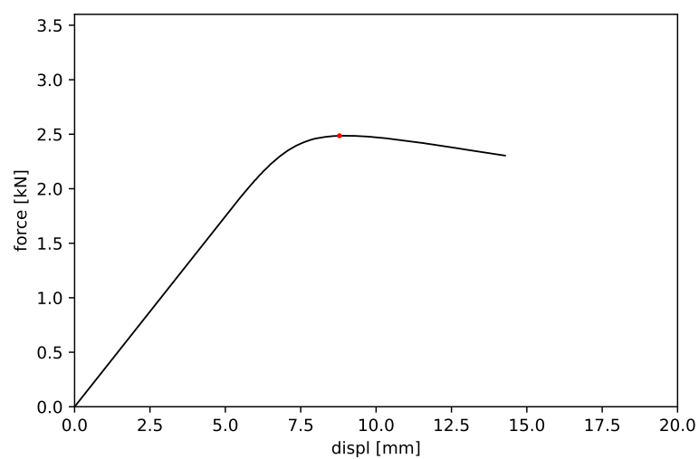
Obrázek 28: Vzorek č. 28 - maximální síla 2.486 kN a příslušný posun 8.784 mm
