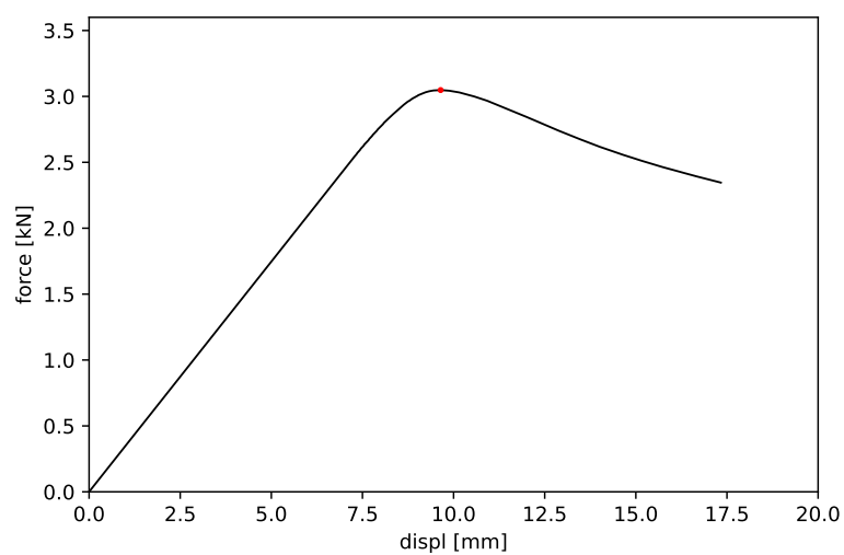
Obrázek 36: Vzorek č. 36 - maximální síla 3.048 kN a příslušný posun 9.645 mm
