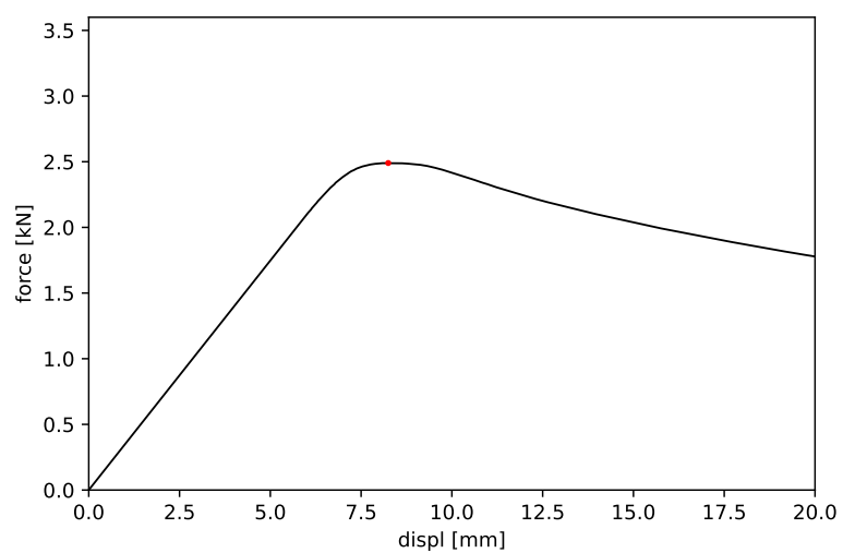
Obrázek 16: Vzorek č. 16 - maximální síla 2.490 kN a příslušný posun 8.247 mm
