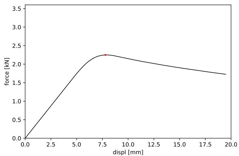
Obrázek 3: Vzorek č. 3 - maximální síla 2.249 kN a příslušný posun 7.791 mm
