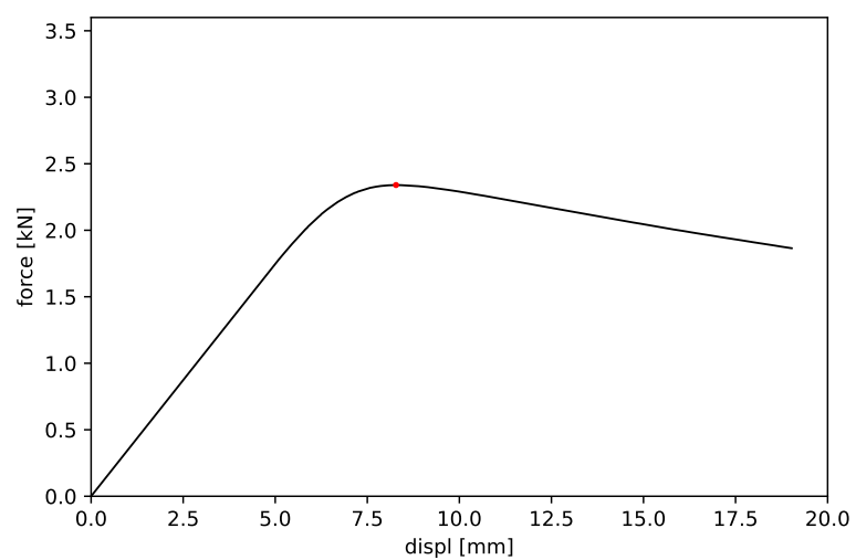
Obrázek 7: Vzorek č. 7 - maximální síla 2.340 kN a příslušný posun 8.280 mm
