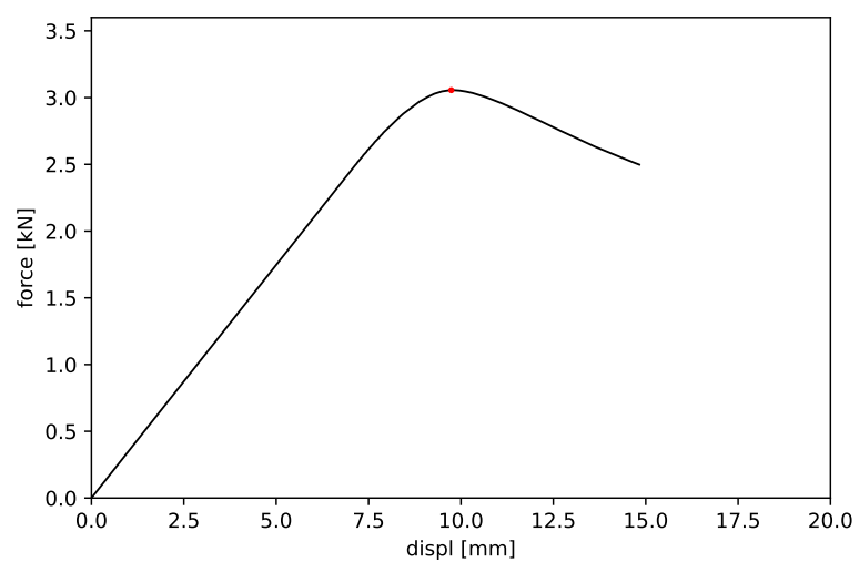
Obrázek 52: Vzorek č. 52 - maximální síla 3.056 kN a příslušný posun 9.739 mm
