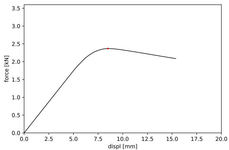
Obrázek 32: Vzorek č. 32 - maximální síla 2.369 kN a příslušný posun 8.484 mm
