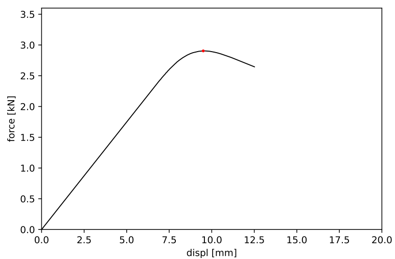
Obrázek 55: Vzorek č. 55 - maximální síla 2.904 kN a příslušný posun 9.501 mm
