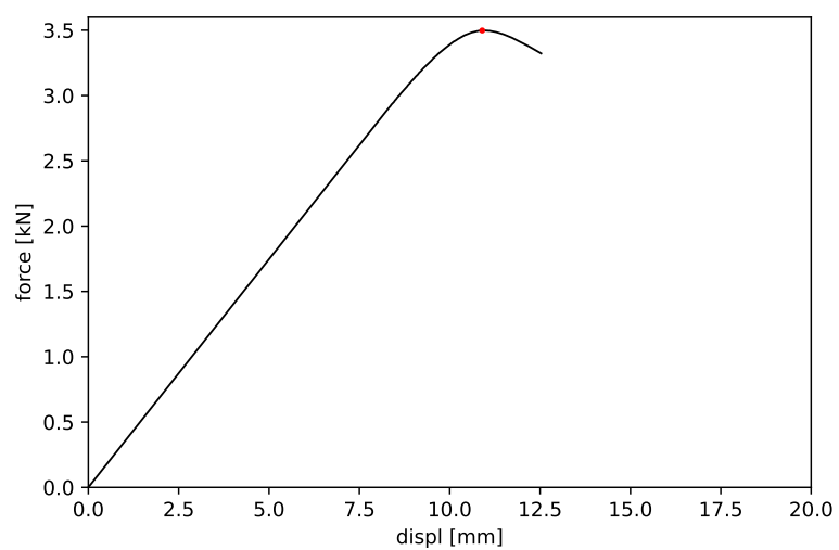
Obrázek 63: Vzorek č. 63 - maximální síla 3.498 kN a příslušný posun 10.899 mm
