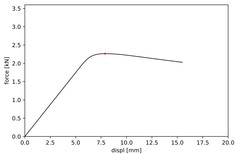
Obrázek 26: Vzorek č. 26 - maximální síla 2.266 kN a příslušný posun 7.898 mm
