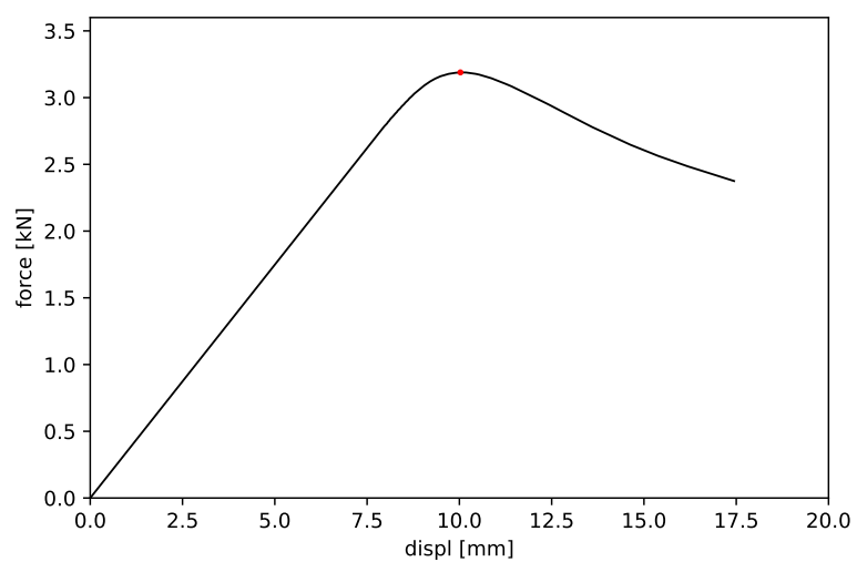
Obrázek 59: Vzorek č. 59 - maximální síla 3.189 kN a příslušný posun 10.028 mm
