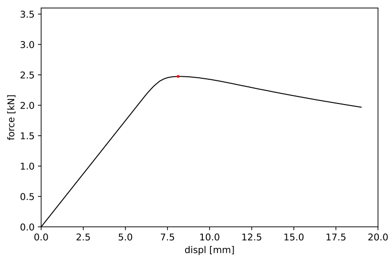
Obrázek 39: Vzorek č. 39 - maximální síla 2.474 kN a příslušný posun 8.134 mm
