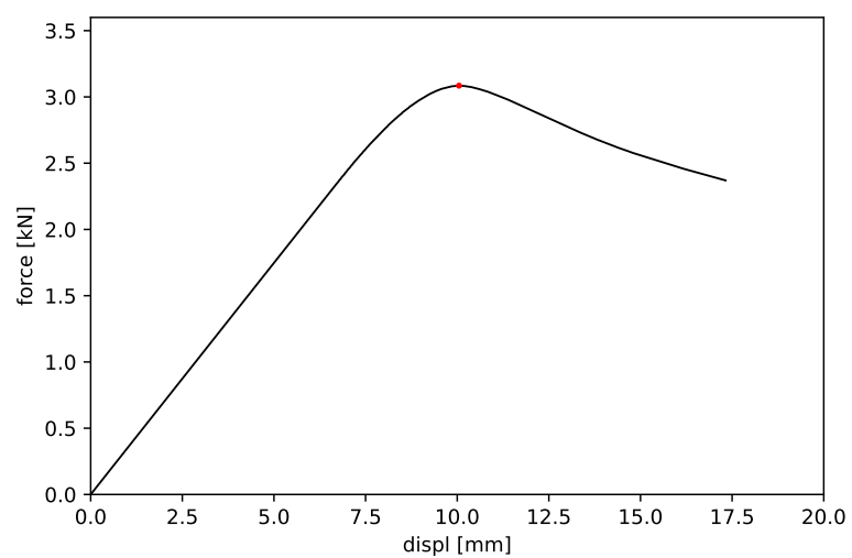
Obrázek 24: Vzorek č. 24 - maximální síla 3.085 kN a příslušný posun 10.049 mm
