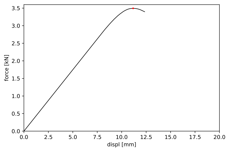
Obrázek 45: Vzorek č. 45 - maximální síla 3.494 kN a příslušný posun 11.167 mm
