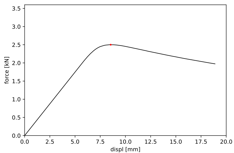
Obrázek 47: Vzorek č. 47 - maximální síla 2.501 kN a příslušný posun 8.537 mm
