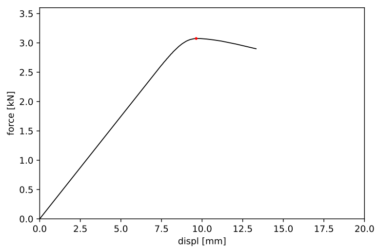
Obrázek 38: Vzorek č. 38 - maximální síla 3.075 kN a příslušný posun 9.637 mm
