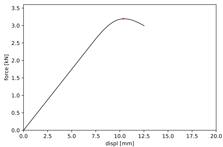
Obrázek 54: Vzorek č. 54 - maximální síla 3.193 kN a příslušný posun 10.351 mm
